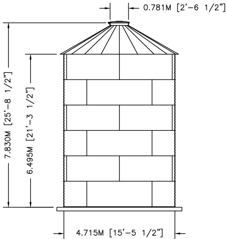
ELEVATION
